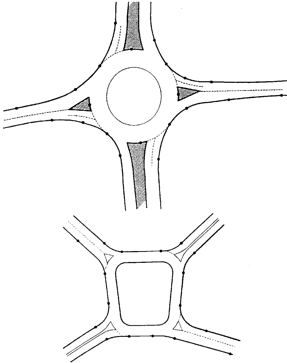
شکل ۷-۴- مثالهایی از میادین واقع در تقاطعهای چهار راه
