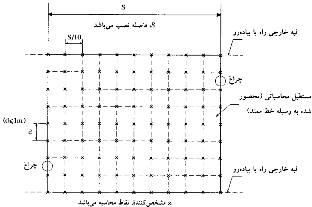
شکل ۱-۵- تشکیل "مستطیل محاسباتی" و "نقاط محاسبه" داخل آن، به منظور محاسبه شدت روشنایی راههای محلی
