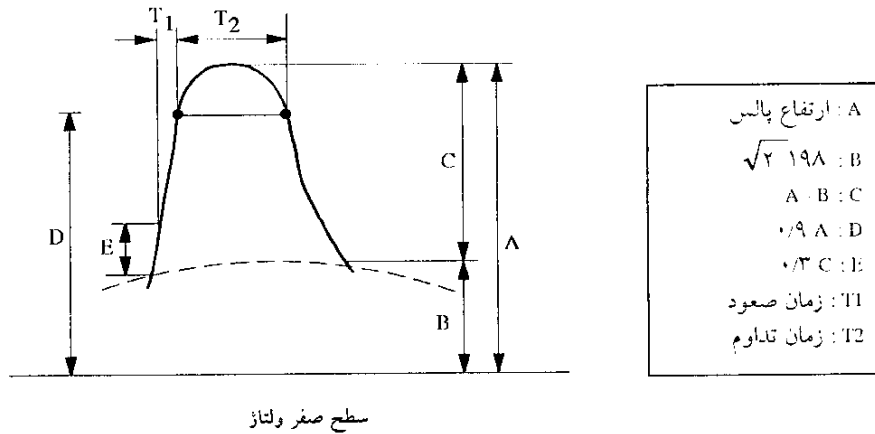
شکل ۱-۱۲- شکل موج پالس ولتاژ راه انداز لامپهای بخار سدیم پرفشار
