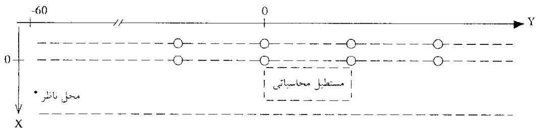
شکل ۳-۹- آرایش نصب در وسط
