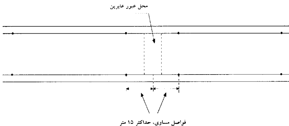
شکل ۳-۲۳- وضعیت استقرار پایه‌ها در اطراف محل عبور عابرین در روش نصب رویرو
