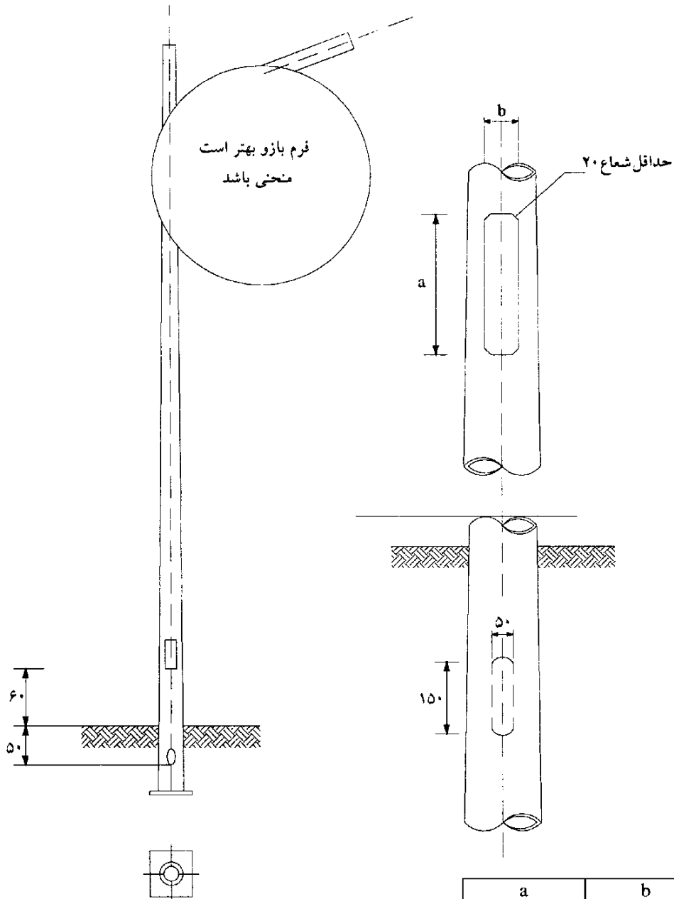
شکل ۱۳-۵- موقعیت محل جعبه فیوز و کابل ورودی به پایه (ابعاد به میلیمتر)
