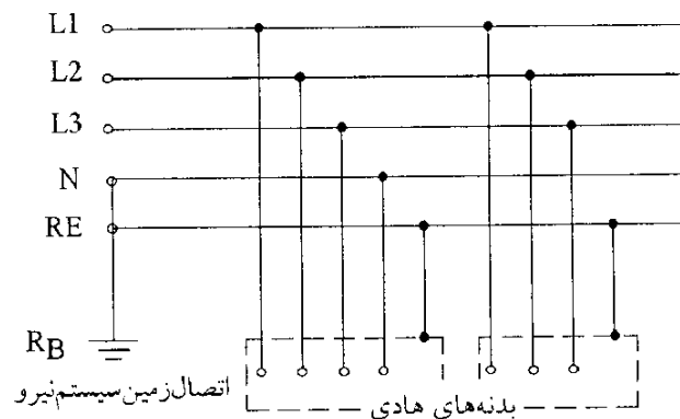
شکل ۴-۱۴- سیستم زمین نوع TN-S
