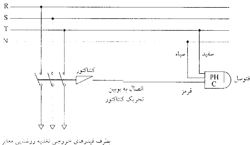
شکل ۱۴-۷- دیاگرام مدار فرمان روشنایی معابر با استفاده از کنتاکتور
