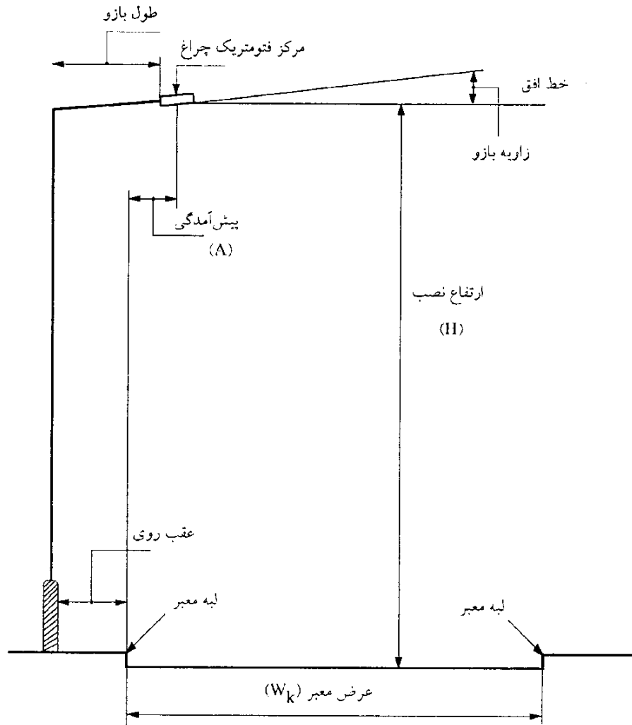
شکل ۱-۱- مشخصات قسمتهای مختلف پایه
