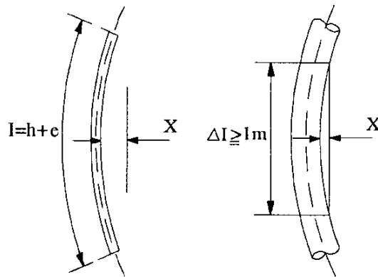
شکل ۹-۱۳- تغییر مکان پایه از حالت عمودی
