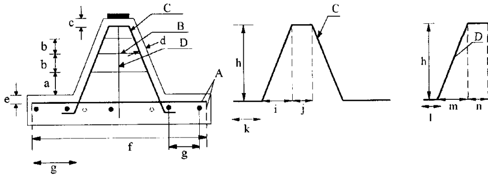
شکل ۱۳-۱۵- آرماتورهای فونداسیونها
