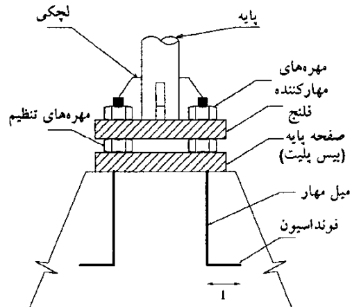
شکل ۱۳-۱۷- طریقه نصب پایه بر روی فونداسیون
