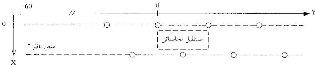
شکل ۳-۸- آرایش نصب زیگزاگ
