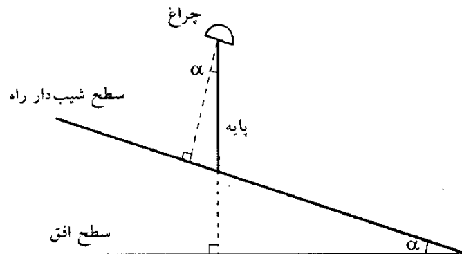
شکل ۳-۱۹- روش نصب چراغ در شیبها
