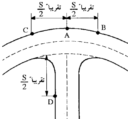
شکل ۶-۷-ب- روشنایی تقاطعها در انحنای راه
