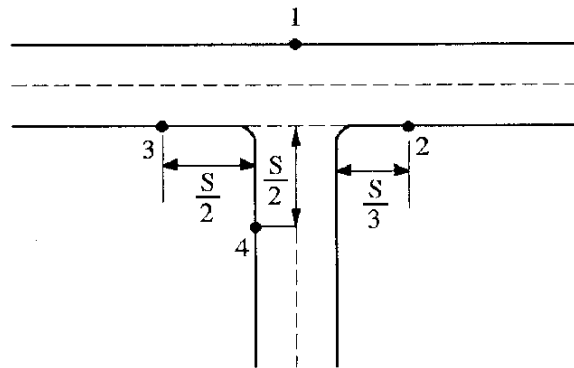
شکل ۶-۱- سیستم روشنایی تقاطع T
