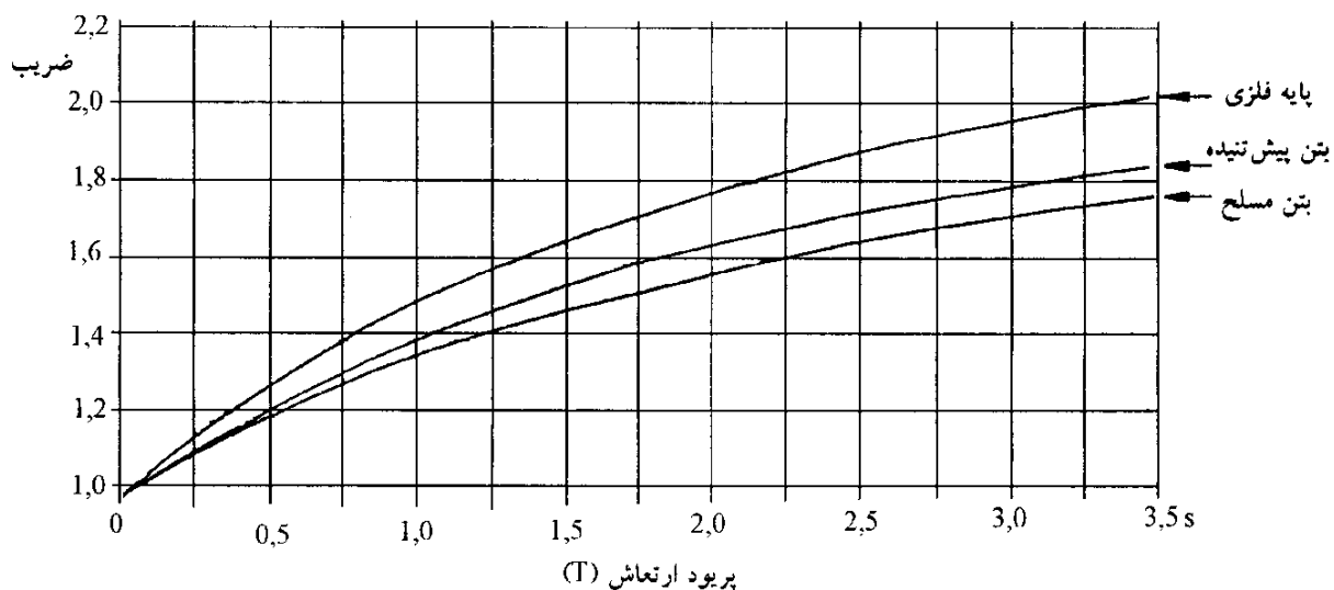
شکل ۱۳-۱- ضریب \beta برحسب پریود ارتعاش پایه
