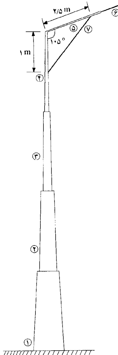
شکل ۱۳-۱۰- شماره قطعات مختلف پایه
