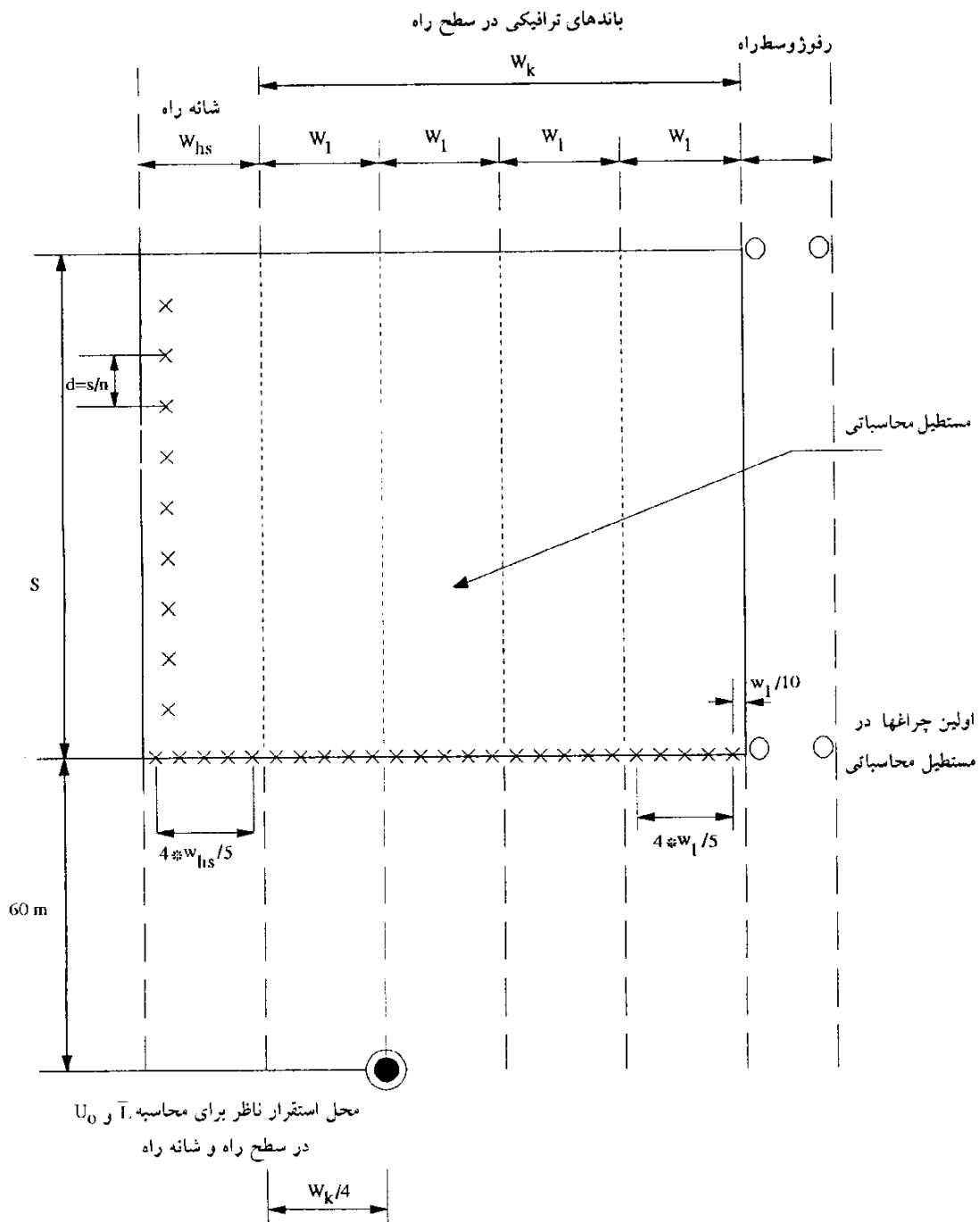
شکل ۴-۲- موقعیت "نقاط محاسبه" و محل استقرار ناظر، با توجه به محل نصب چراغها در یک راه شریانی درجه ۱ چهارباندی (در هر طرف راه) با آرایش نصب در وسط (X، مشخص کننده هر نقطه محاسبه می باشد)
