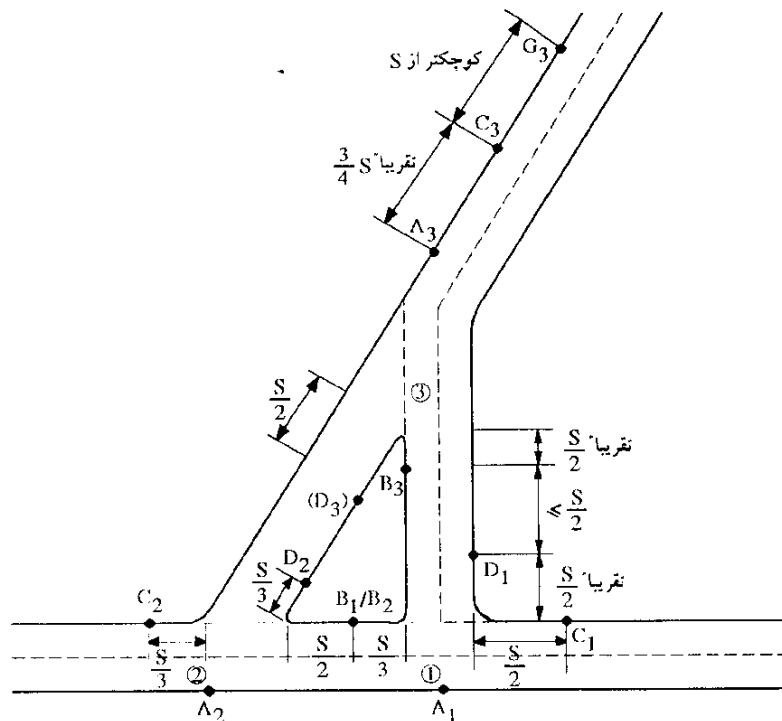
شکل ۶-۶-الف- تقاطع با جزیره ترافیکی مثلثی
