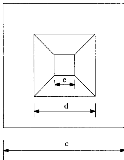
شکل ۱۳-۱۴- ابعاد فونداسیونها
