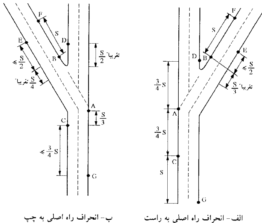
شکل ۶-۵- سیستم روشنایی تقاطعهای چنگالی
