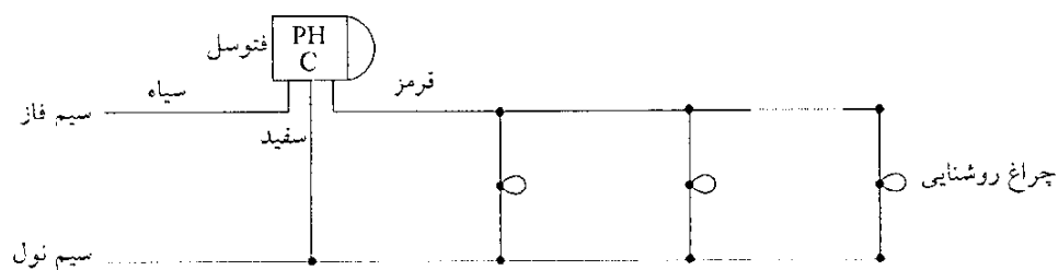
شکل ۶-۱۴- دیاگرام مدار فرمان تعدادی چراغ روشنایی به کمک عملکرد مستقیم فتوسل
