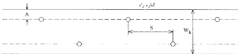
شکل ۱-۳- آرایش نصب زیگزاگ چراغهای روشنایی معابر
