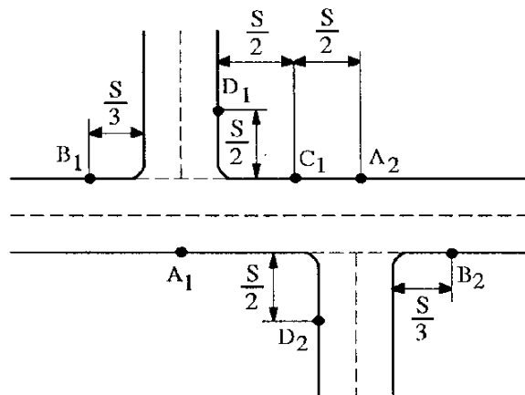
شکل ۲-۶- سیستم روشنایی تقاطعهای زیگزآگ
