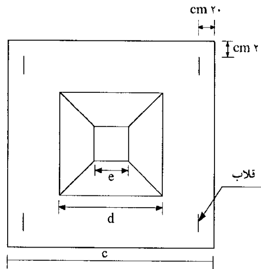
شکل ۱۳-۱۶- محل نصب قلابها
