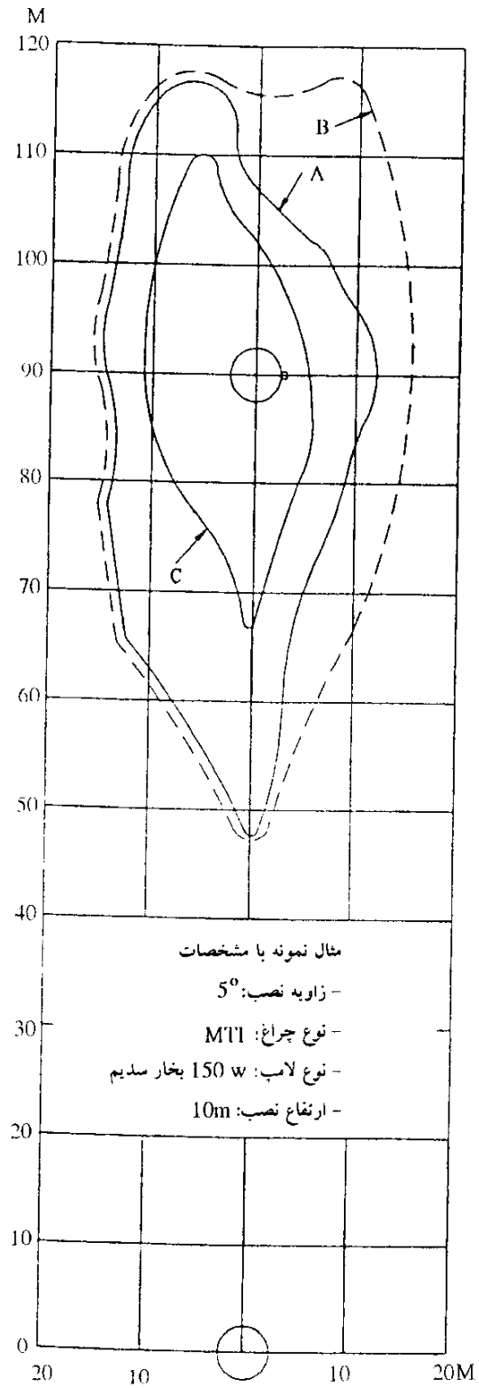
شکل ۳-۱۳- نمونه‌ای از منحنی "درخشندگی ثابت"
