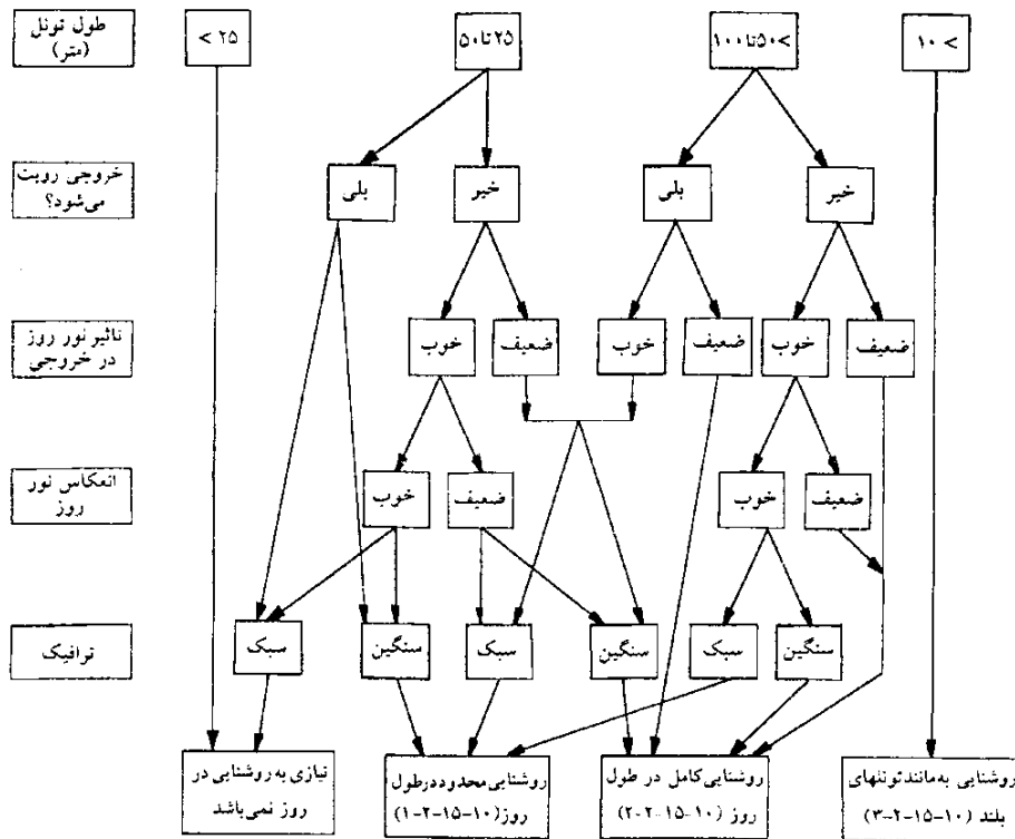
شکل ۱۰-۸- روشنایی تونلهای کوتاه در طول روز
