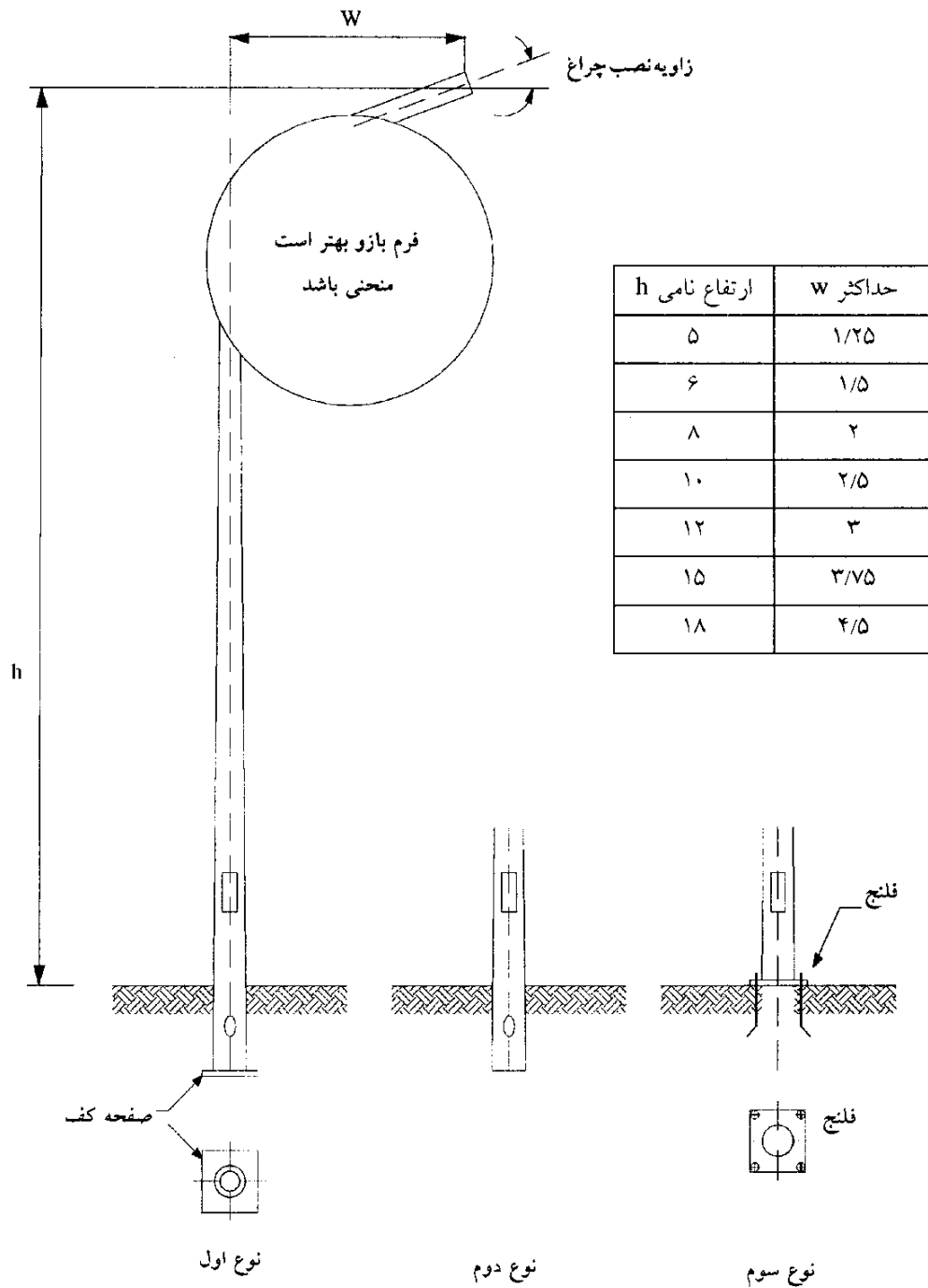
شکل ۱۳-۴- ابعاد اصلی پایه‌های دارای بازو (متر)
