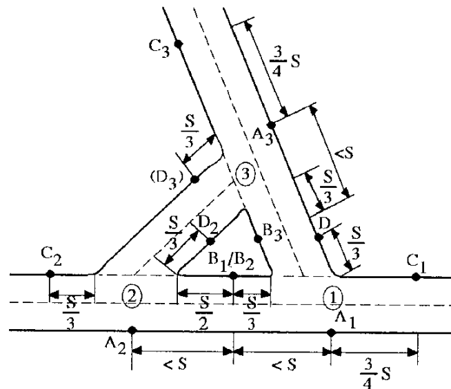
شکل ۶-۶-ب- تقاطع با جزیره ترافیکی مثلثی
