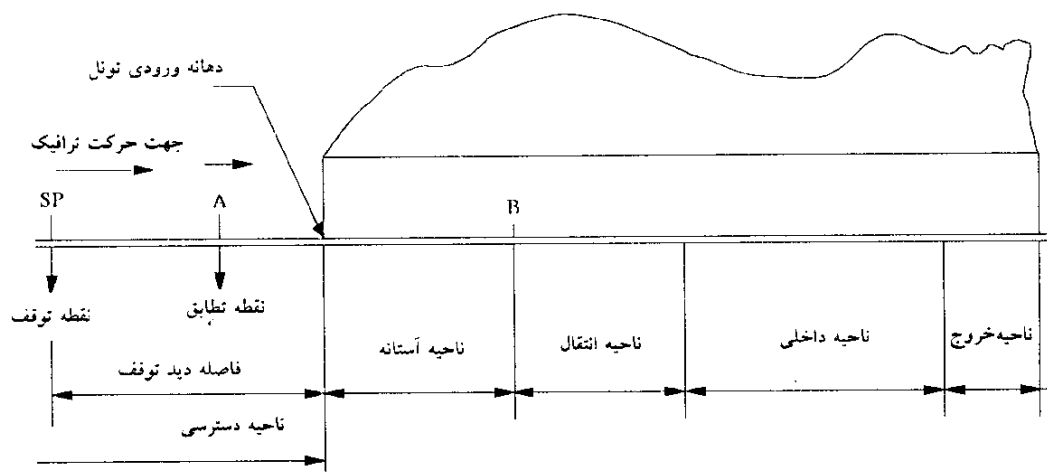
شکل ۱۰-۱- مقطع طولی از یک تونل واقع در راه بکطرفه
