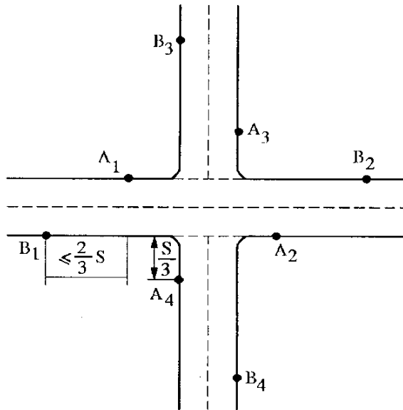
شکل ۶-۳- سیستم روشنایی چهارراهها
