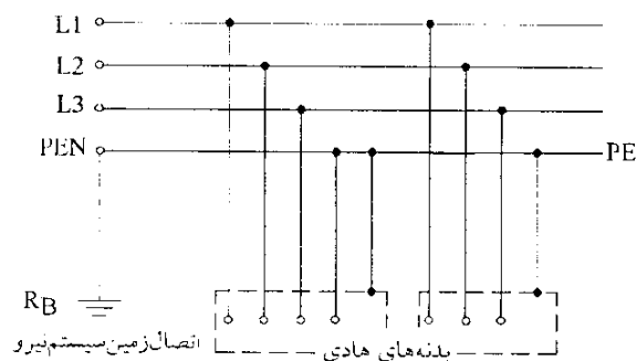
شکل ۵-۱۴- سیستم زمین نوع TN-C
