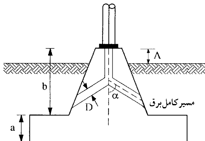
شکل ۱۳-۱۳- فونداسیون پایه‌های روشنایی
