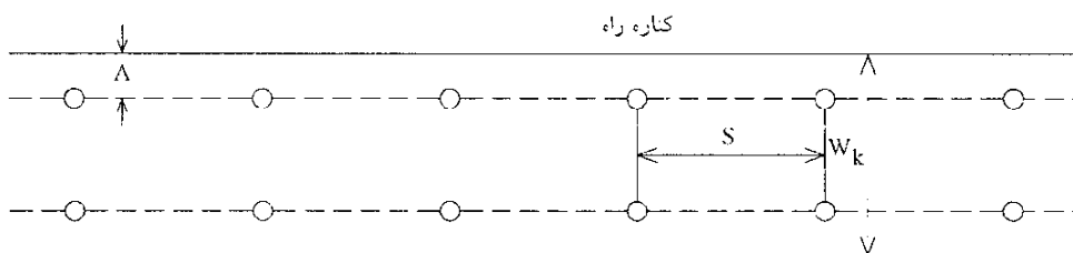
شکل ۲-۳- آرایش نصب روبرو چراغهای روشنایی معابر
