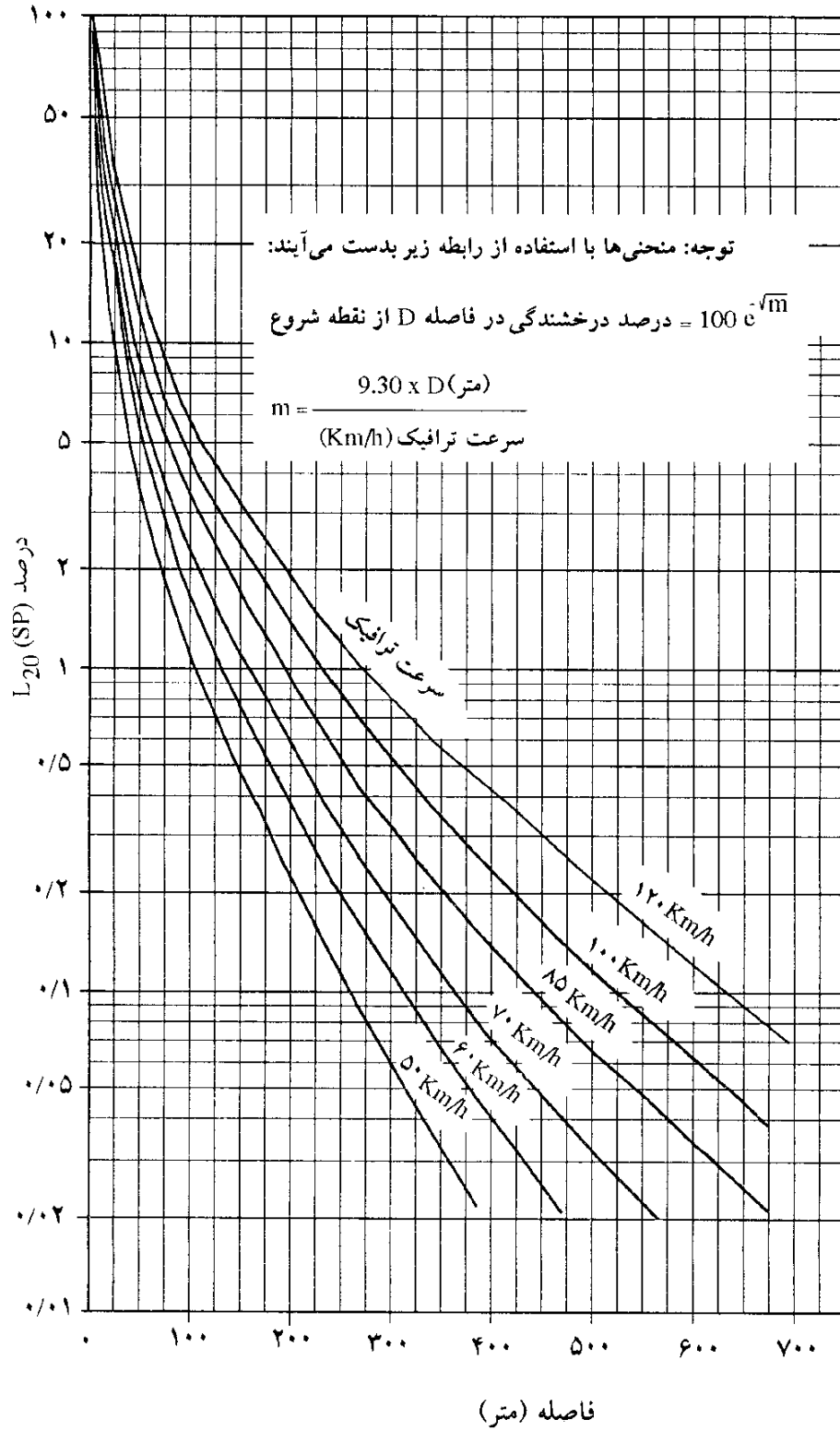
شکل ۱۰-۳- منحنیهای کاهش درخشندگی در ناحیه انتقال
