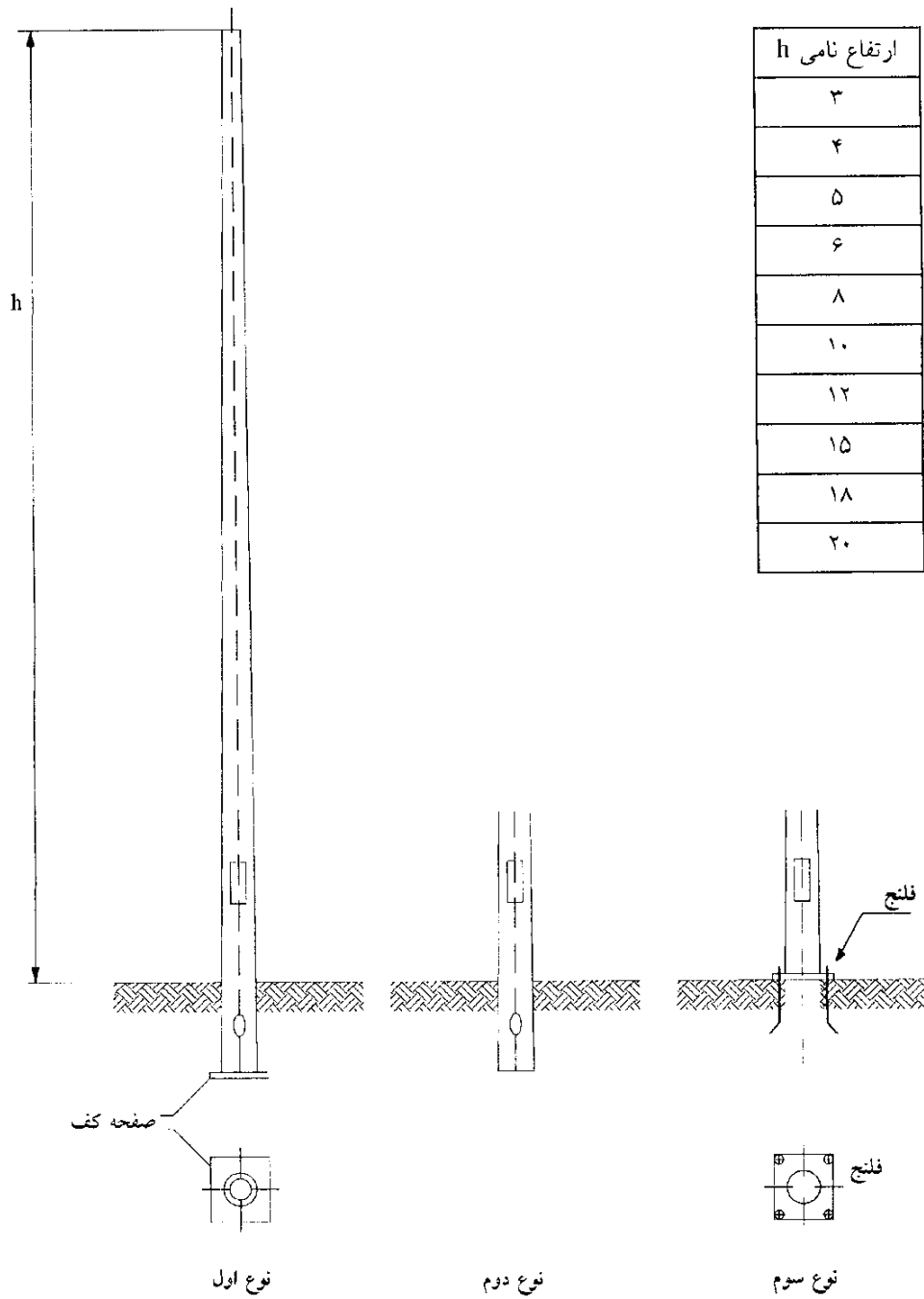
شکل ۱۳-۳- ابعاد اصلی پایه‌های بدون بازو (متر)
